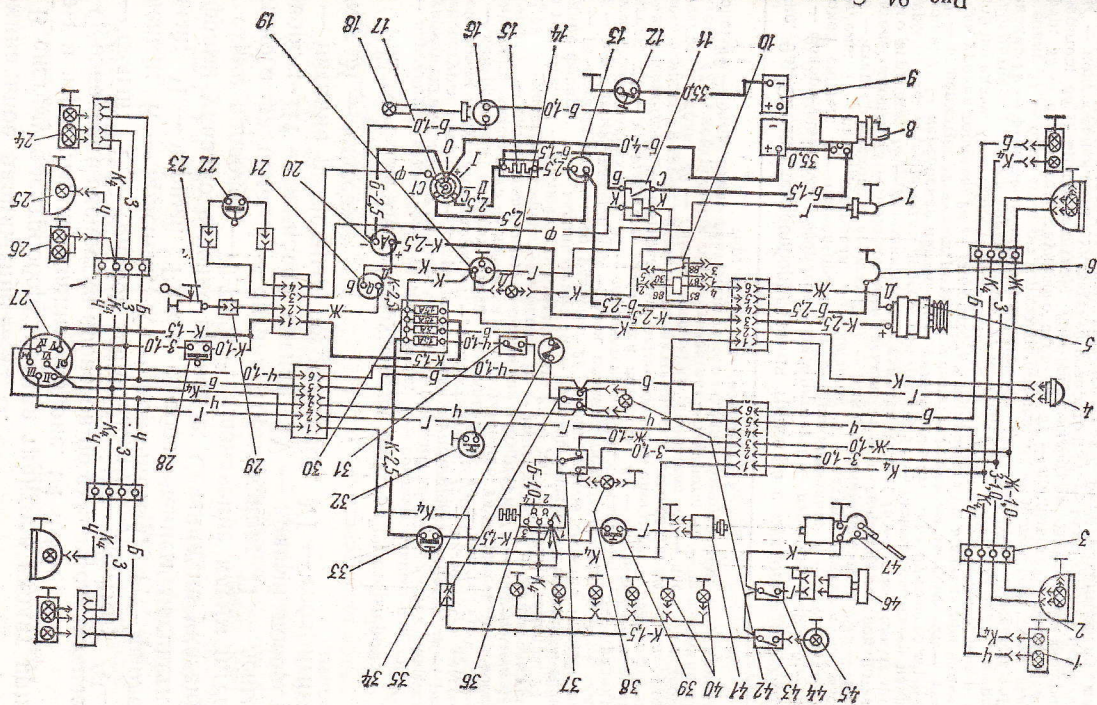
Рис. 94. Схема электрооборудования трактора со стартером (см. стр. 305)
