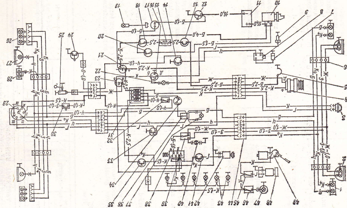
Рис. 95. Схема электрооборудования трактора с пусковым аппаратом (см. стр. 305)
